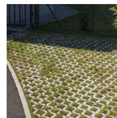
Dalle alvéolaire
